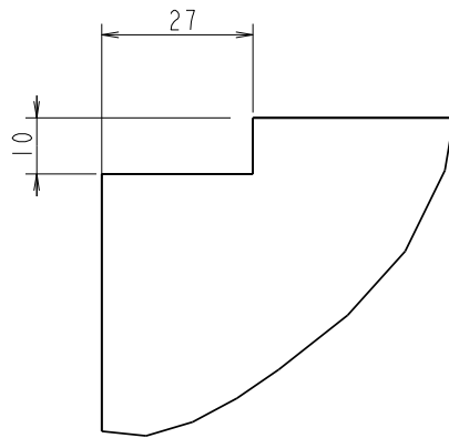
DETAIL A ECHELLE 1,000 4 découpes identiques
