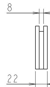
TRaverse LONGITUDINALE DECOUPEE REF F2004.12_CAJ.008
